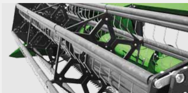
HASPELZINKENWICKELSCHUTZ Verhindert das Wickeln von Unkräutern (z.B.: Kamille) um die Haspelzinkenrohre
