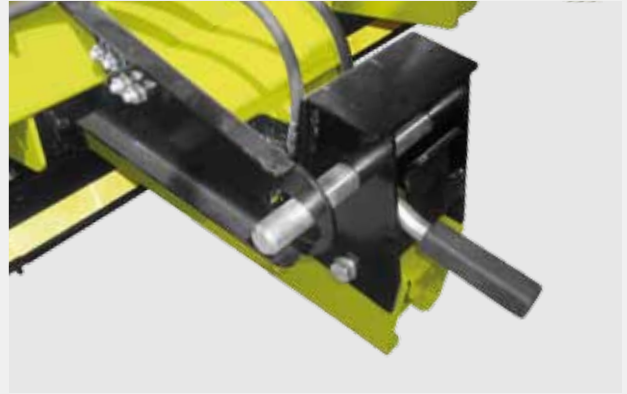
EINFACH ZU BETÄTIGENDE, SICHERE VERRIEGELUNG Mit großen Toleranzen beim An- und Abhängen des Schneidwerkes
